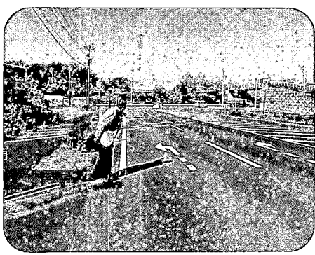
⑪ 県道新設: 菊陽町との境・道明付近
