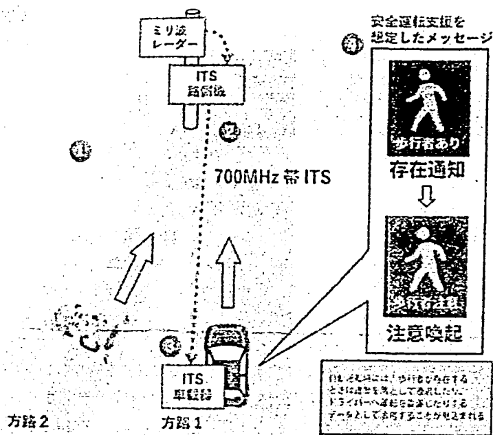
▲図2：ミリ波レーダーを用いた実証実験 出典：関西電力、パナソニック、ゼロ・サム、トヨタIT開発センター報道資料「自動運転社会を見据えた路車間通信に関する技術実証の実施について」(2019)
