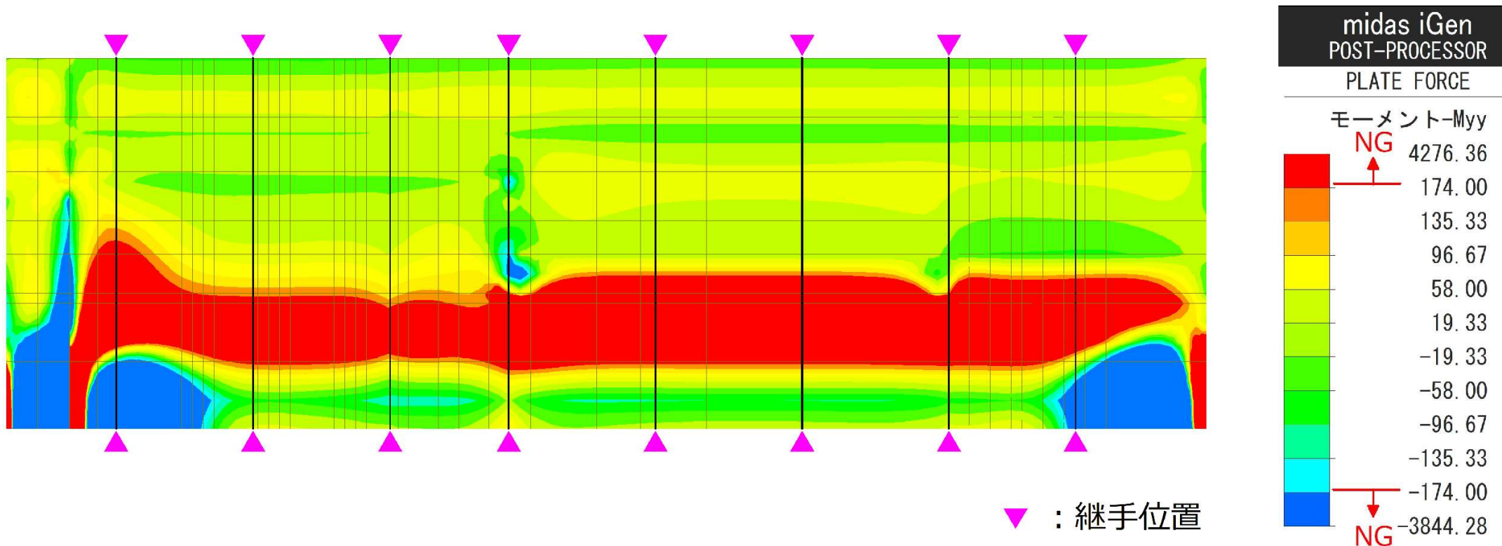
応力図(西面)
