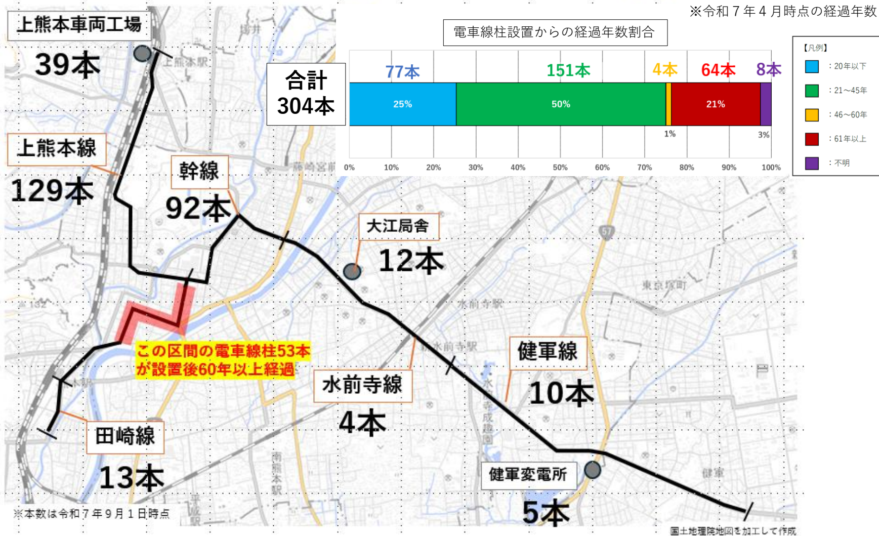
交通局所有の電車線柱 分布図
