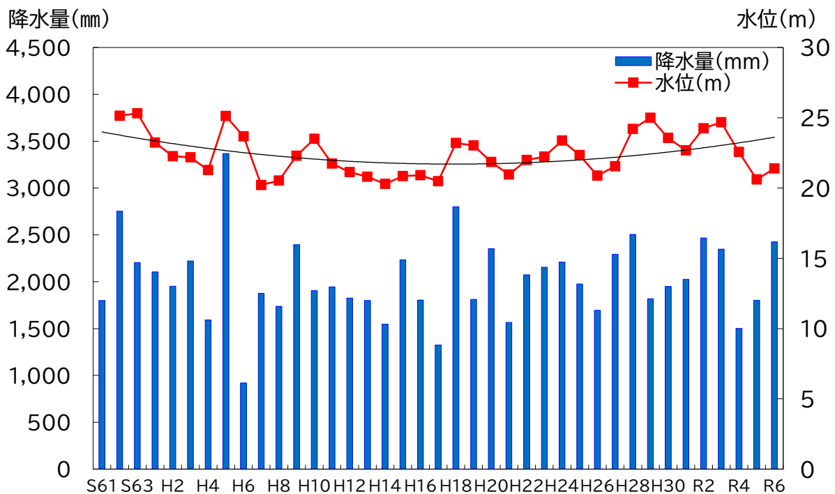
地下水位の経年変化(日向東観測井[戸島地区])
