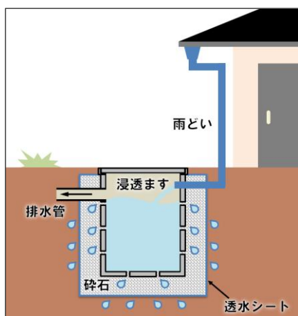
雨水浸透ます イメージ
